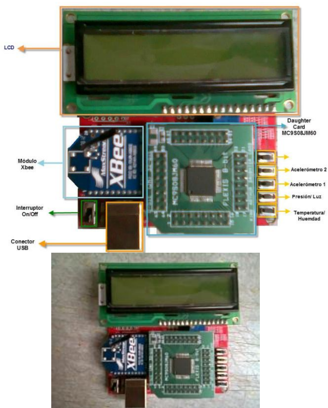
Fig. 5. Diseño final del coordinador.
