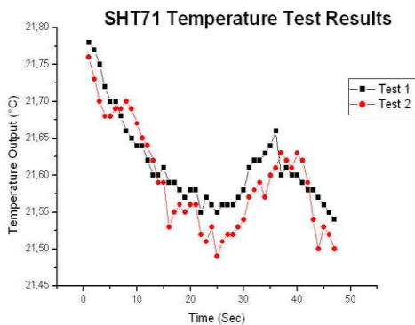
Fig. 8. Resultados experimentales de temperatura obtenidos del sensor SHT71.
