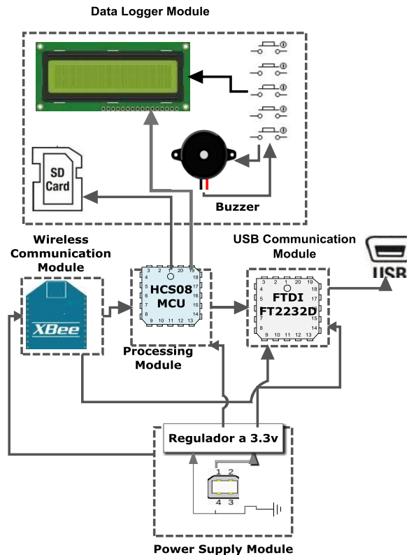
Fig. 4. Diagrama de bloques del coordinador.
