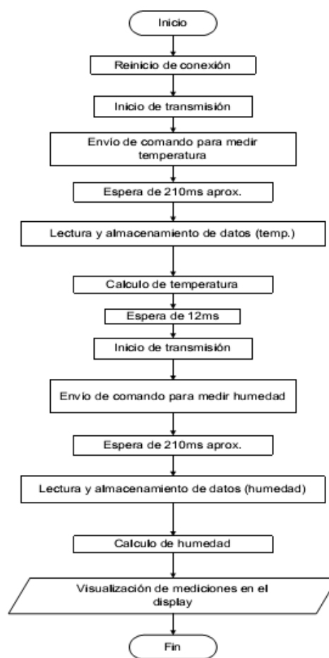
Fig 6. Diagrama de flujo de las secuencias para obtener medidas del sensor SHT71
