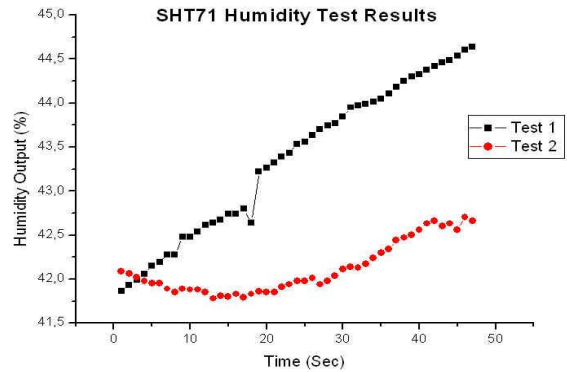
Fig. 9. Resultados experimentales de humedad relativa obtenidos del sensor SHT71.
