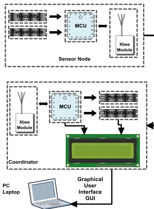
Fig. 1. Diagrama esquemático del sistema de monitoreo inalámbrico.
