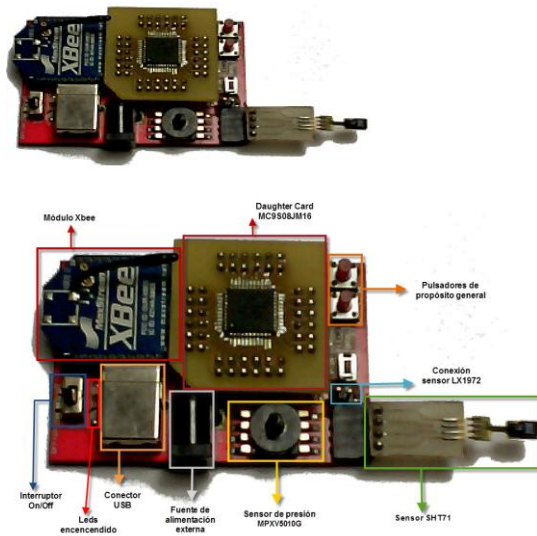
Fig. 3. Diseño final del nodo sensor.
