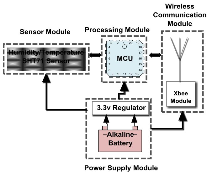
Fig. 2 . Diagrama de bloques del nodo sensor.
